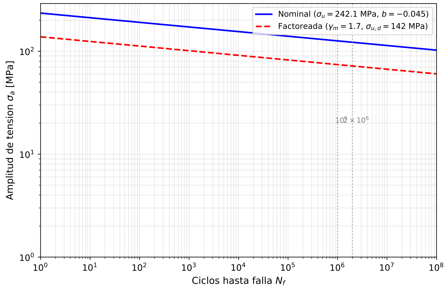
Curva S-N del GFRP \pm 45^\circ (infusion al vacio)
